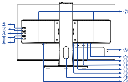
<Вид сзади>
