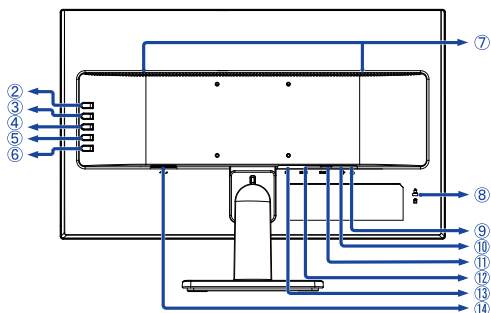
<Вид сзади>
