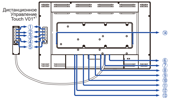
<Вид сзади>
